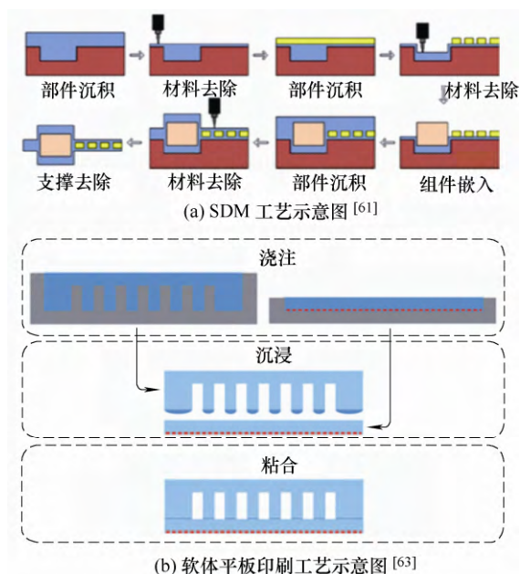
图 4 SDM 和软体平板印刷工艺
