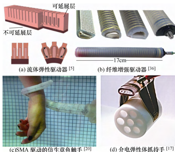
图 1 几种软体机器人仿生结构
