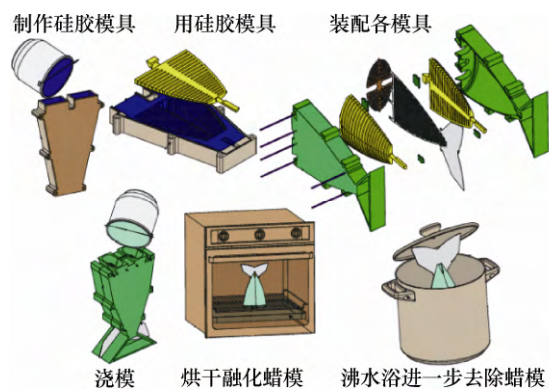
图 5 失蜡铸造工艺示意图 [63]
